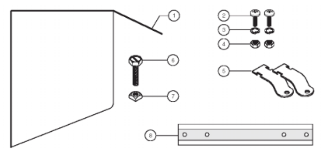
图 3-6 遮阳罩套件
